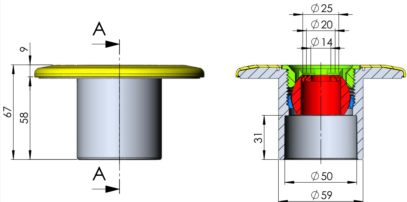
SECCIÓN A-A
